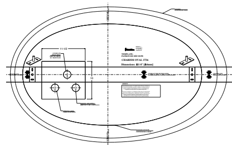
Patron d'installation du Charism Oval 5736
